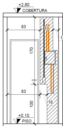
VISTA 2 - CIRCULAÇÃO
