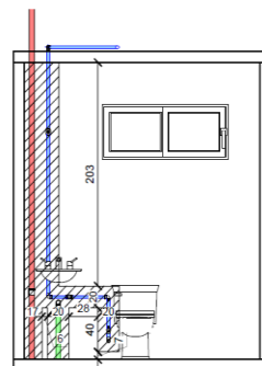
VISTA 3 - WC.
