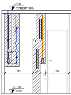
VISTA 1 - WC.
