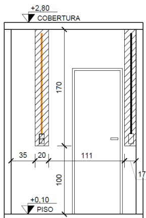
VISTA 1 - CIRCULAÇÃO
