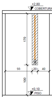
VISTA 2 - WC.
